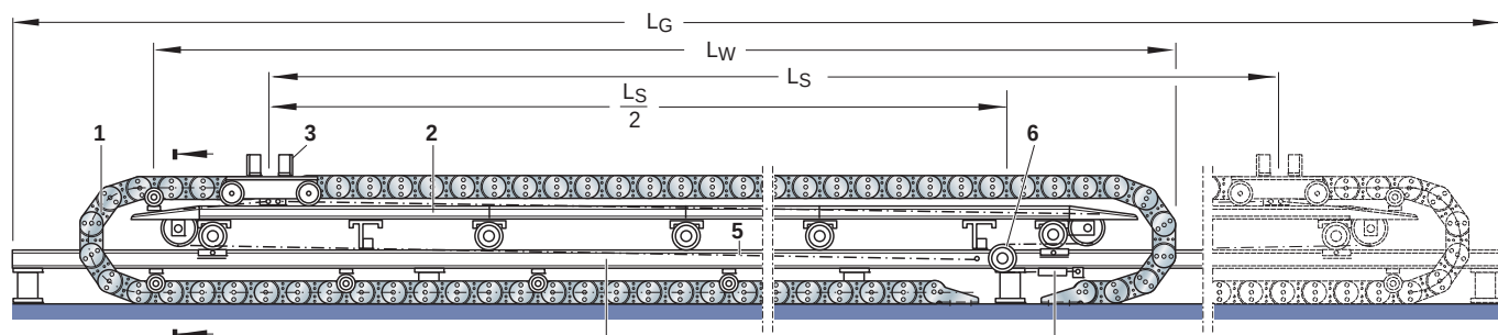
- Disposizione contrapposta (raffigurazione schematica)
