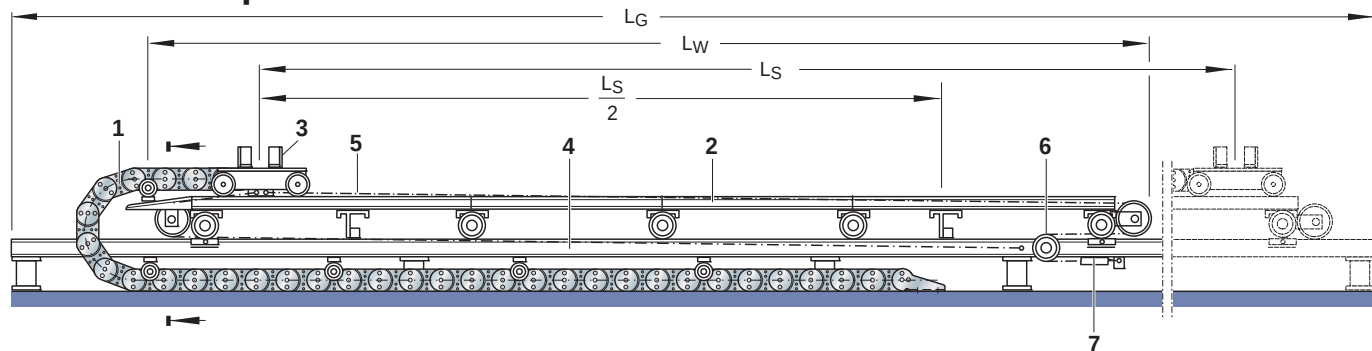
- Disposizione semplice (raffigurazione schematica)
