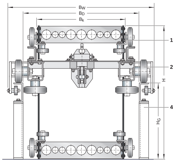
Sezione dell'installazione
